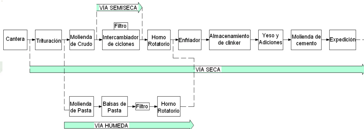
Figura 4. Diagrama de flujo del proceso de fabricación del cemento
